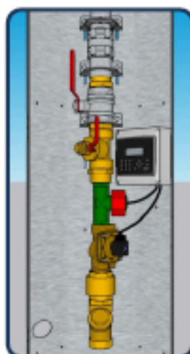
Compteur programmable avec automate
